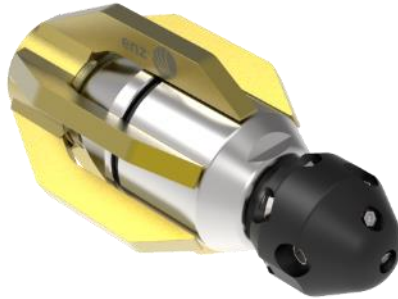
Abbildung 5: Bulldog® 406.037xx
